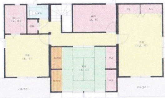
〈2F平面図〉
