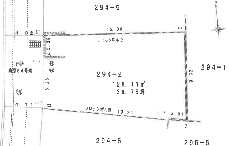
現況図 1/200
