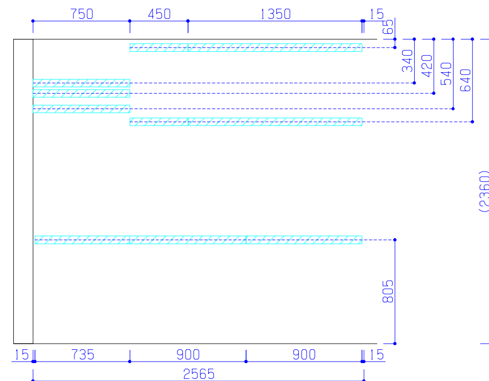
栈木展開図A
