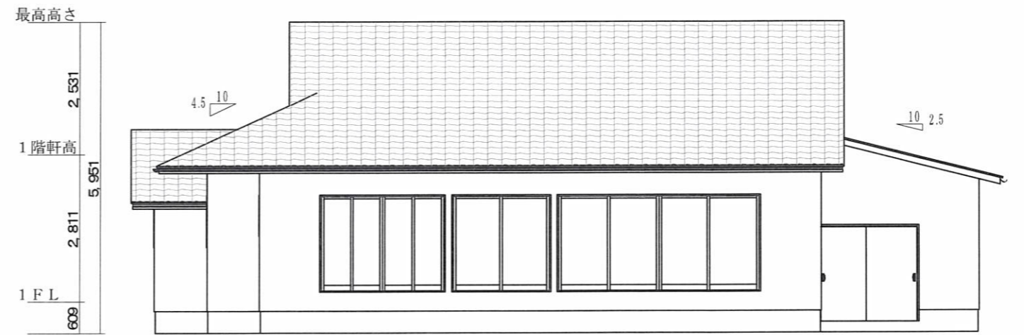
北側立面図
