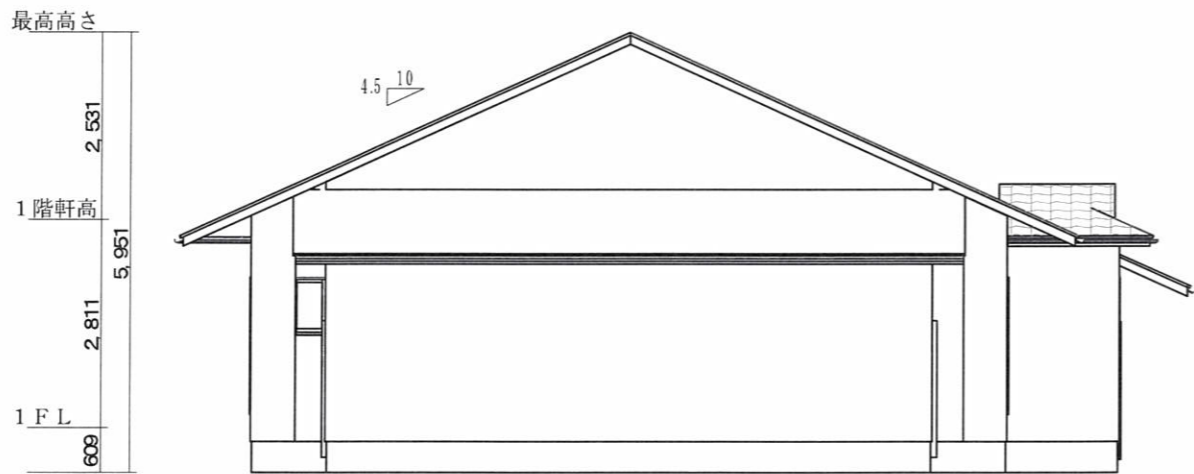
西側立面図
