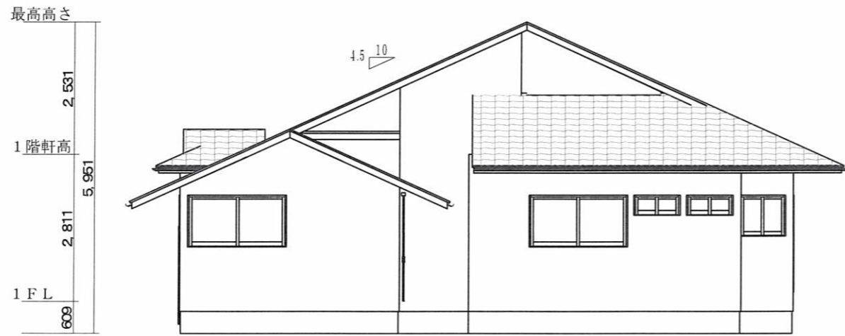
東側立面図
