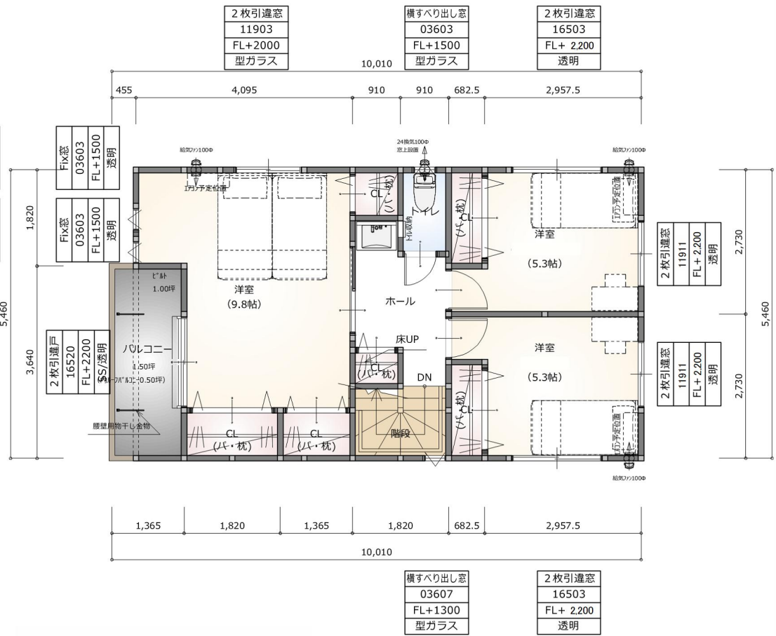
2階平面図
