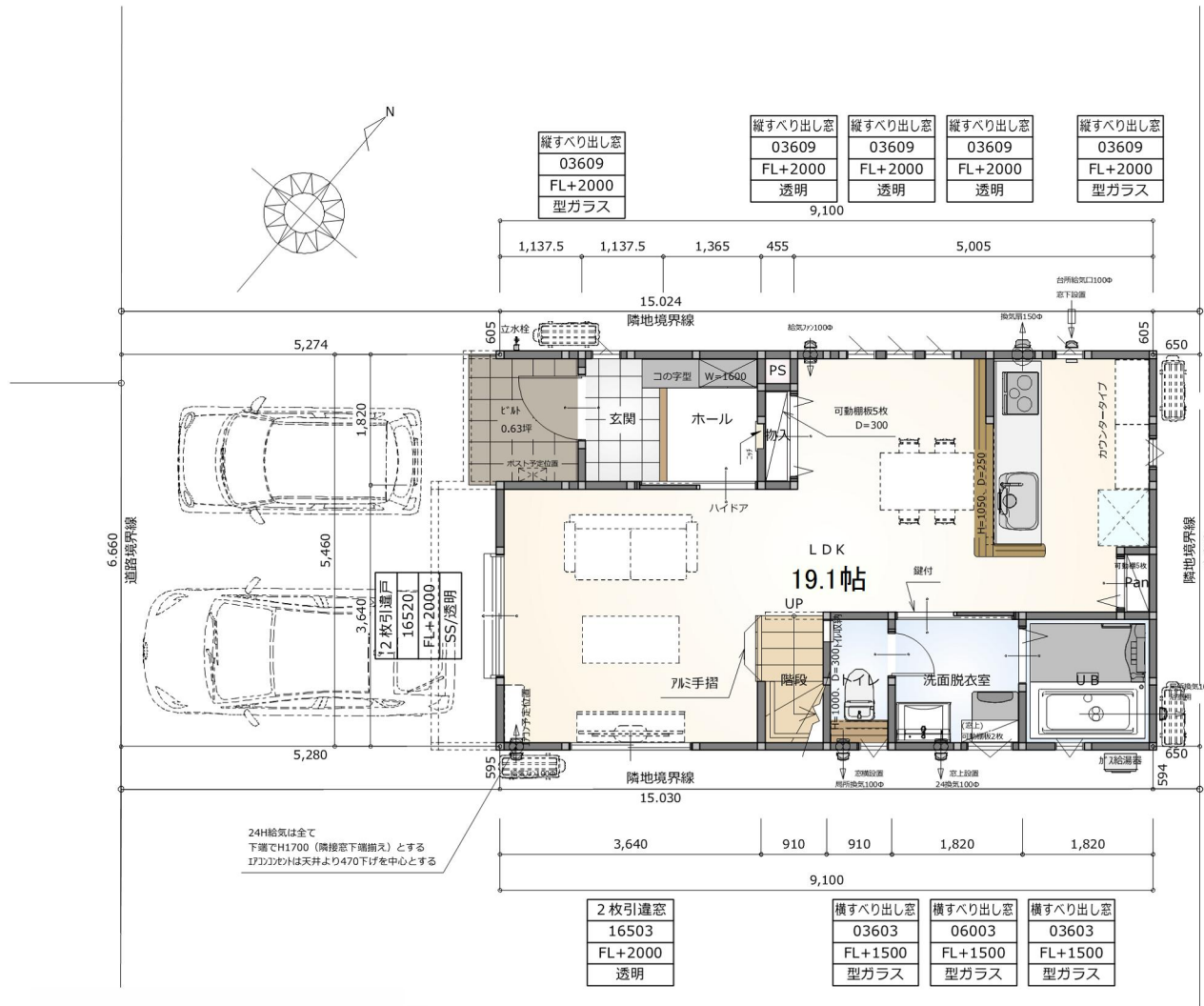
1階平面図
