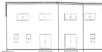
南側立面
